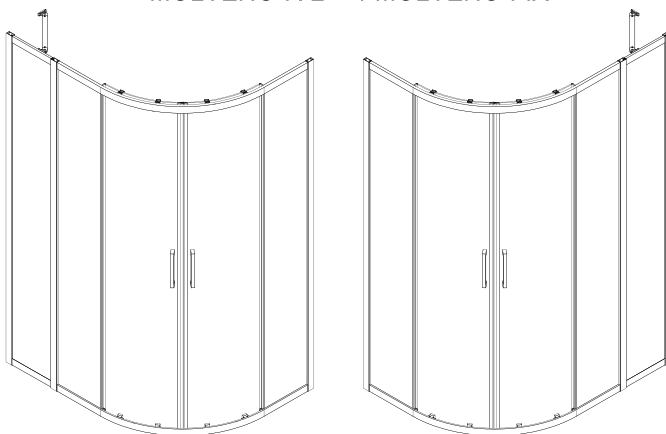
MOLVENO-R-2 + 1 MOLVENO-FIX
