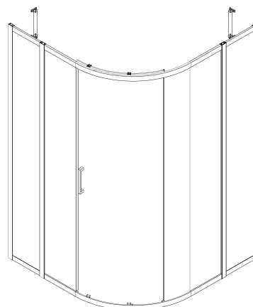
MOLVENO-A-2 + 2 MOLVENO-FIX
