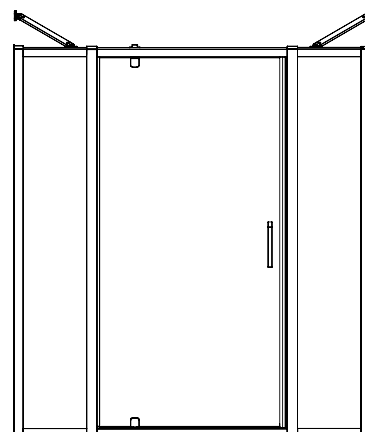
MOLVENO-BA-1 + 2 MOLVENO-FIX
